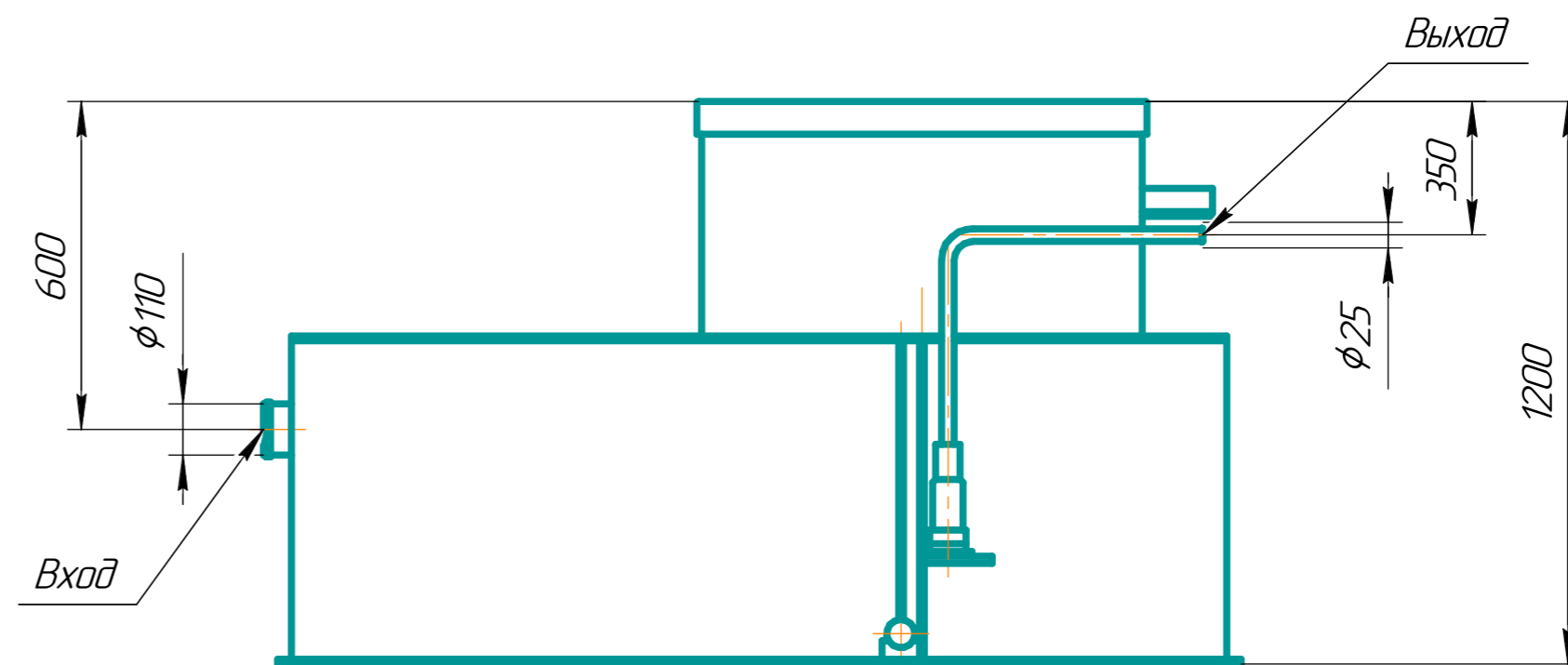
В-В
