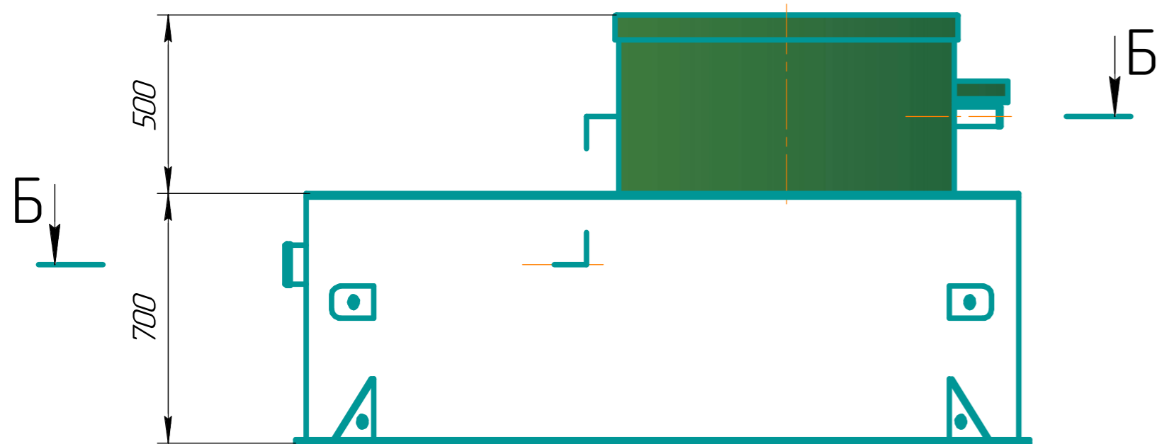
Вид спереди
